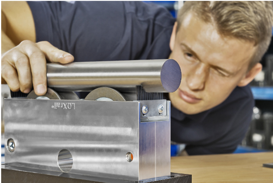
Bild: LOXrail-Systeme sind mit massiven Schienenwellen aus Präzisions- oder Edelstahl in Durchmessern von 25 mm und 40 mm erhältlich
